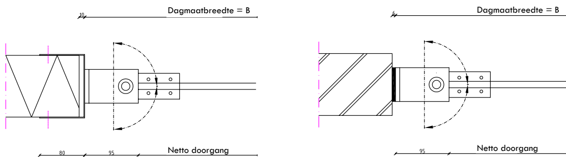
Wandomvattend kozijn
