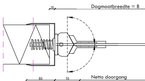
Wandomvattend kozijn, type 8
