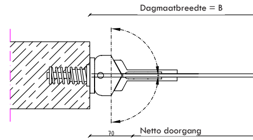
Montage direct in houten kozijn
