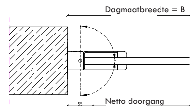
Montage direct in houten kozijn
