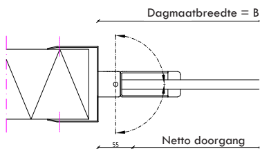
Wandomvattend RVS kozijn
