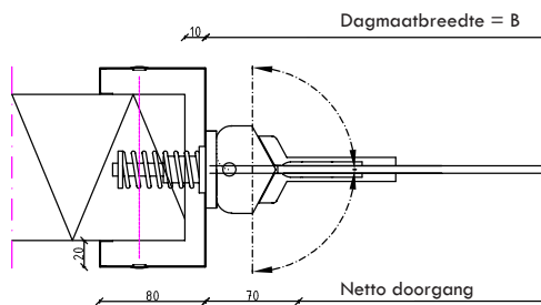
Wandomvattend kozijn, type 7
